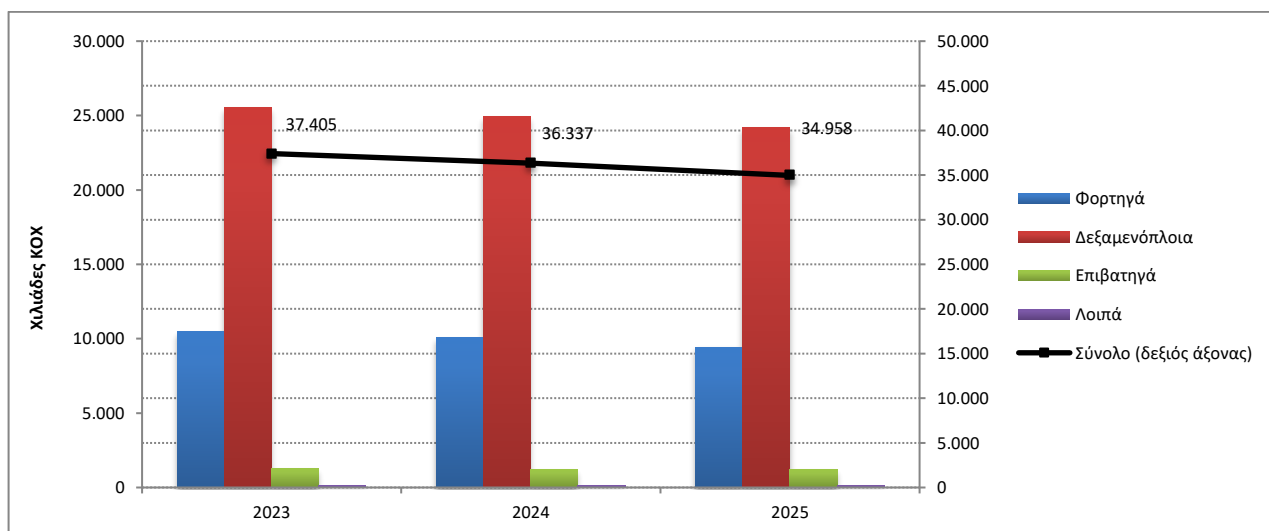
Γράφημα 2β: Χωρητικότητα των ελληνικών εμπορικών πλοίων 100 ΚΟΧ και άνω, κατά κατηγορίες πλοίων, Σεπτέμβριος 2023 – 2025
