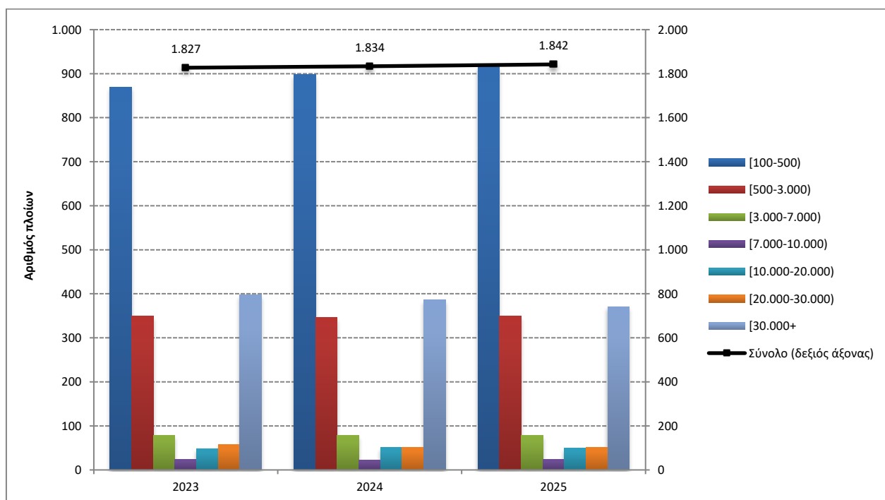
Γράφημα 3: Κατανομή των ελληνικών εμπορικών πλοίων 100 ΚΟΧ και άνω, κλιμάκια ολικής χωρητικότητας, Σεπτέμβριος 2023 – 2025
