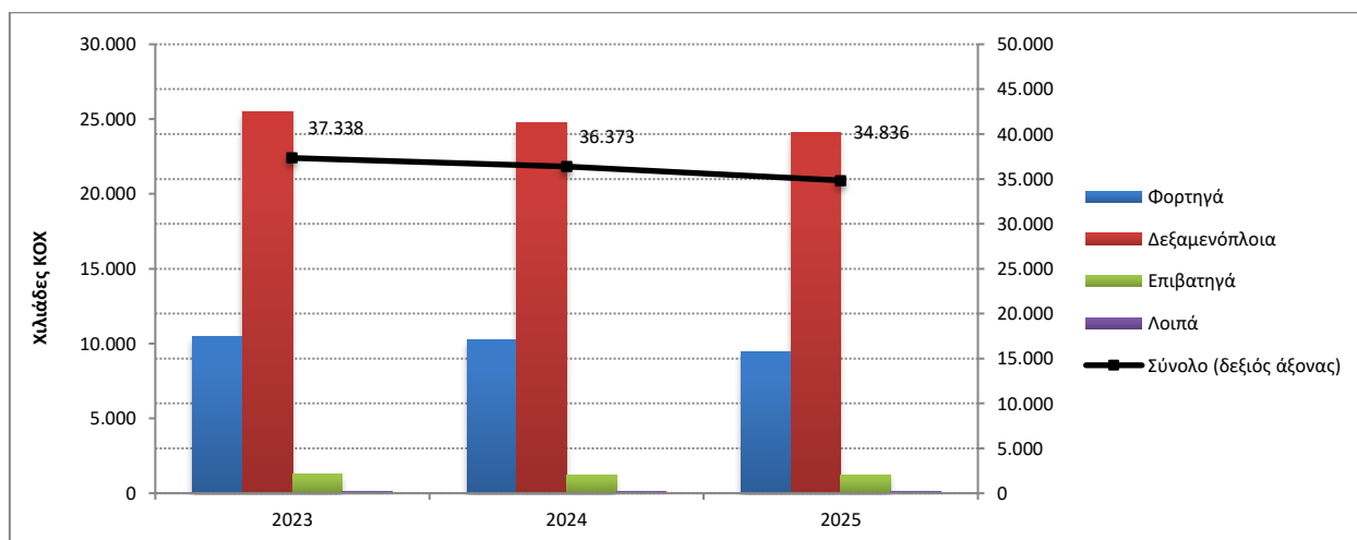
Γράφημα 2β: Χωρητικότητα των ελληνικών εμπορικών πλοίων 100 ΚΟΧ και άνω, κατά κατηγορίες πλοίων, Αύγουστος 2023 – 2025
