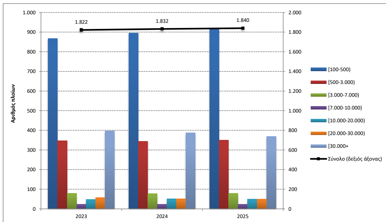
Γράφημα 3: Κατανομή των ελληνικών εμπορικών πλοίων 100 ΚΟΧ και άνω, κλιμάκια ολικής χωρητικότητας, Αύγουστος 2023 – 2025
