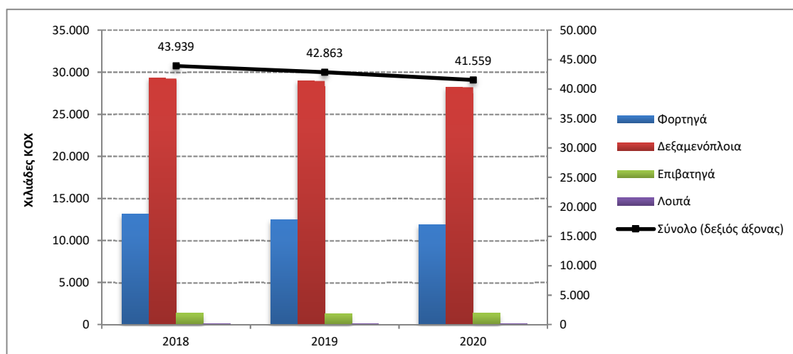
Γράφημα 2β: Χωρητικότητα των ελληνικών εμπορικών πλοίων 100 ΚΟΧ και άνω, κατά κατηγορίες πλοίων, Μάιος 2018 – 2020
