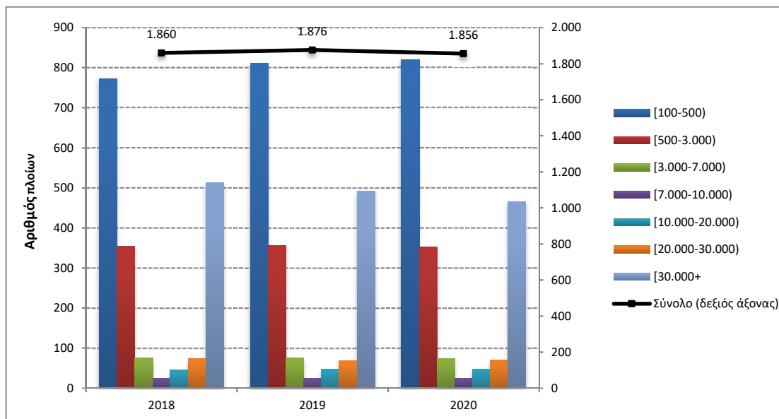
Γράφημα 3: Κατανομή των ελληνικών εμπορικών πλοίων 100 ΚΟΧ και άνω, κατά κλιμάκια ολικής χωρητικότητας, Μάιος 2018 – 2020
