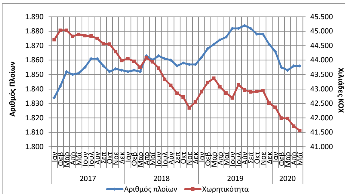
Γράφημα 1: Δύναμη και Ολική Χωρητικότητα των ελληνικών εμπορικών πλοίων 100 ΚΟΧ και άνω, σε μηνιαία βάση, Ιανουάριος 2017 – Μάιος 2020
