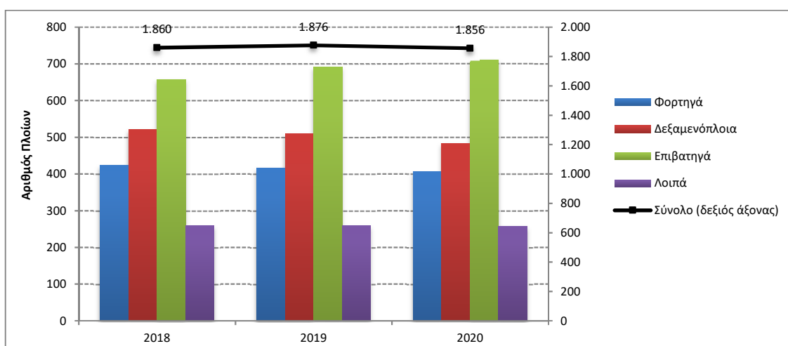
Γράφημα 2α: Δύναμη των ελληνικών εμπορικών πλοίων 100 ΚΟΧ και άνω, κατά κατηγορίες πλοίων, Μάιος 2018 – 2020
