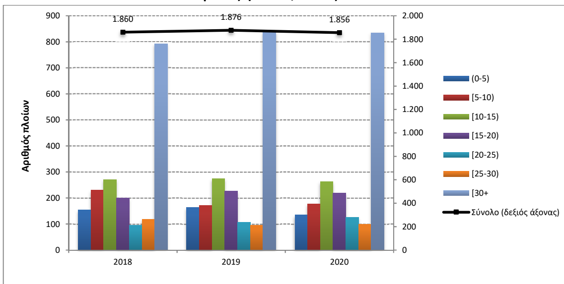
Γράφημα 4α: Κατανομή των ελληνικών εμπορικών πλοίων 100 ΚΟΧ και άνω, κατά ομάδες ηλικιών, Μάϊος 2018 – 2020
