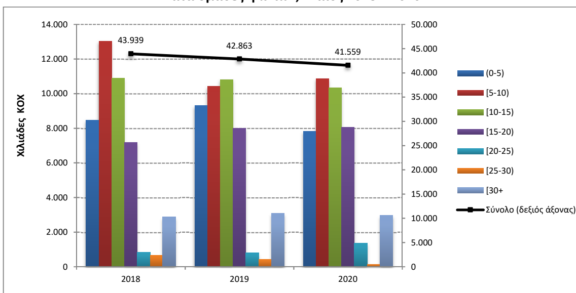
Γράφημα 4β: Κατανομή χωρητικότητας των ελληνικών εμπορικών πλοίων 100 ΚΟΧ και άνω, κατά ομάδες ηλικιών, Μάϊος 2018 – 2020
