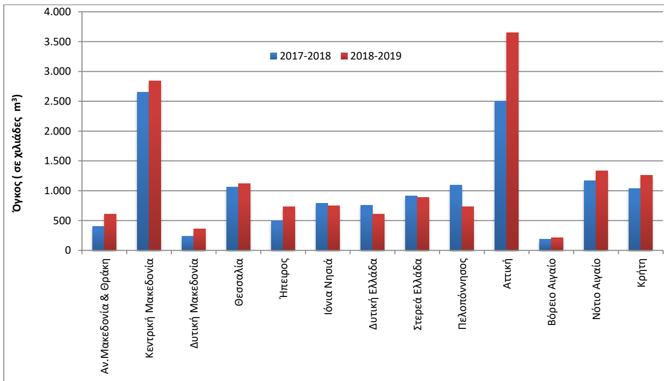
Γράφημα 2. Ιδιωτική Οικοδομική Δραστηριότητα (όγκος), κατά Περιφέρεια, για την περίοδο Σεπτεμβρίου 2017 - Αυγούστου 2018 και Σεπτεμβρίου 2018 - Αυγούστου 2019*
