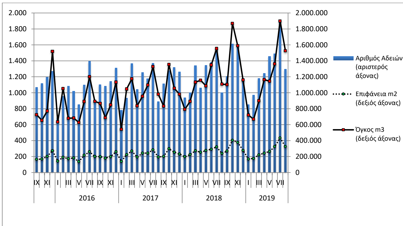
Γράφημα 3. Μηνιαία Ιδιωτική Οικοδομική Δραστηριότητα (Σεπτέμβριος 2015 – Αύγουστος 2019*)
