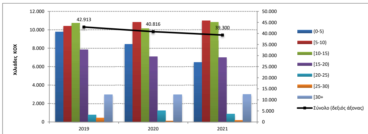
Γράφημα 4β: Κατανομή χωρητικότητας των ελληνικών εμπορικών πλοίων 100 ΚΟΧ και άνω, κατά ομάδες ηλικιών, Οκτώβριος 2019 – 2021
