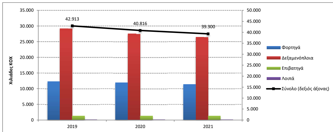
Γράφημα 2β: Χωρητικότητα των ελληνικών εμπορικών πλοίων 100 ΚΟΧ και άνω, κατά κατηγορίες πλοίων, Οκτώβριος 2019 – 2021
