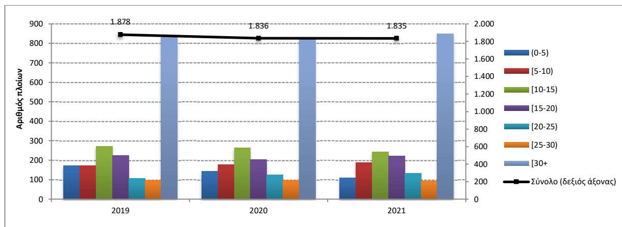
Γράφημα 4α: Κατανομή των ελληνικών εμπορικών πλοίων 100 ΚΟΧ και άνω, κατά ομάδες ηλικιών, Οκτώβριος 2019 – 2021
