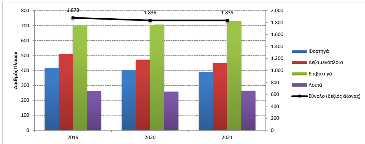
Γράφημα 2α: Δύναμη των ελληνικών εμπορικών πλοίων 100 ΚΟΧ και άνω, κατά κατηγορίες πλοίων, Οκτώβριος 2019 – 2021
