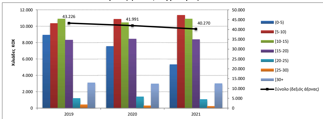
Γράφημα 4β: Κατανομή χωρητικότητας των ελληνικών εμπορικών πλοίων 100 ΚΟΧ και άνω, κατά ομάδες ηλικιών, Φεβρουάριος 2019 – 2021
