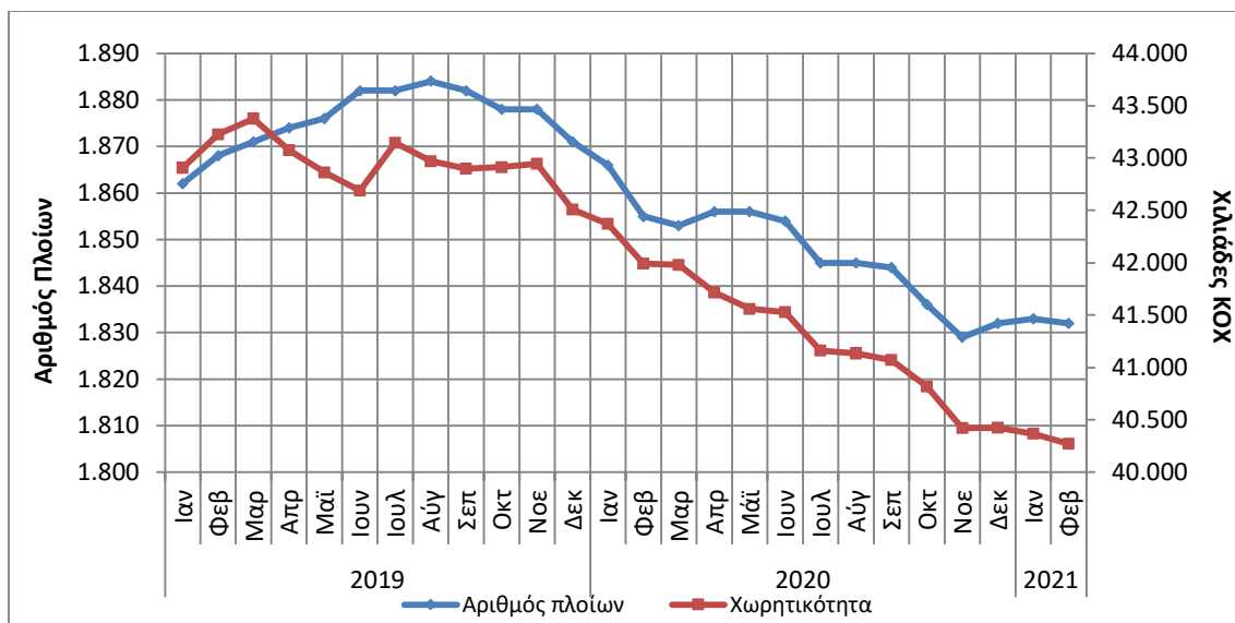
Γράφημα 1: Δύναμη και Ολική Χωρητικότητα των ελληνικών εμπορικών πλοίων 100 ΚΟΧ και άνω, σε μηνιαία βάση, Ιανουάριος 2019 – Φεβρουάριος 2021
