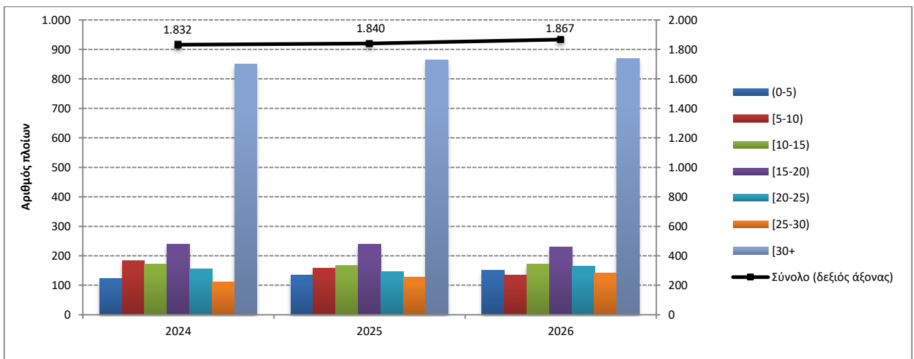
Γράφημα 4α: Κατανομή των ελληνικών εμπορικών πλοίων 100 ΚΟΧ και άνω, κατά ομάδες ηλικιών, Αύγουστος 2024 – 2026
