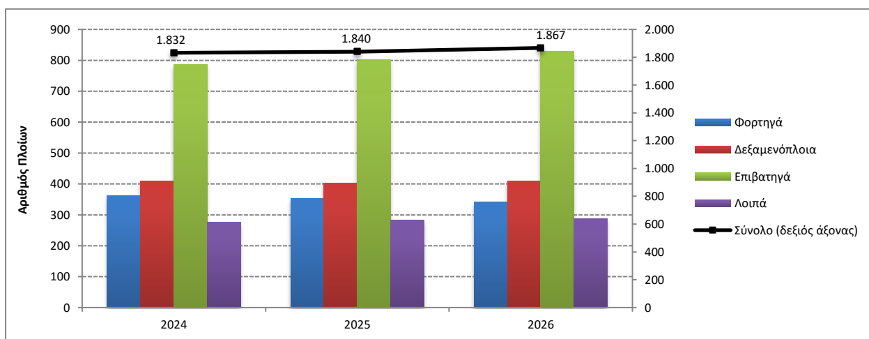
Γράφημα 2α: Δύναμη των ελληνικών εμπορικών πλοίων 100 ΚΟΧ και άνω, κατά κατηγορίες πλοίων Αύγουστος 2024 – 2026
