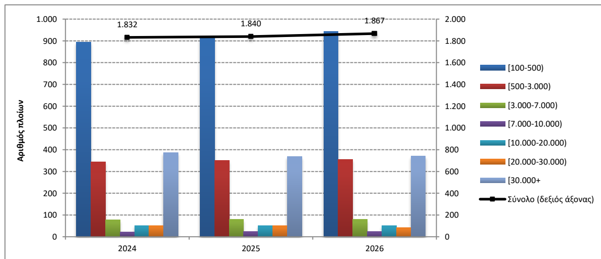
Γράφημα 3: Κατανομή των ελληνικών εμπορικών πλοίων 100 ΚΟΧ και άνω, κλιμάκια ολικής χωρητικότητας, Αύγουστος 2024 – 2026
