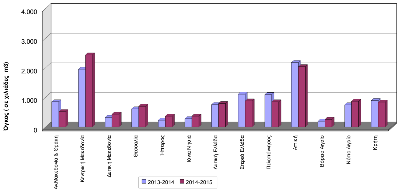
Γράφημα 2. Ιδιωτική Οικοδομική Δραστηριότητα, κατά Περιφέρεια, για την περίοδο Μαρτίου 2013 - Φεβρουαρίου 2014 και Μαρτίου 2014 - Φεβρουαρίου 2015 *
