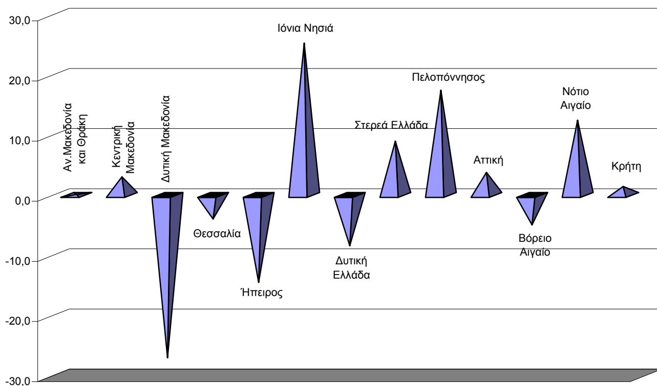
Ιδιωτική Οικοδομική Δραστηριότητα κατά Περιφέρεια Ιανουάριος - Οκτώβριος 2006 και 2005 Μεταβολή % του οικοδομικού όγκου
