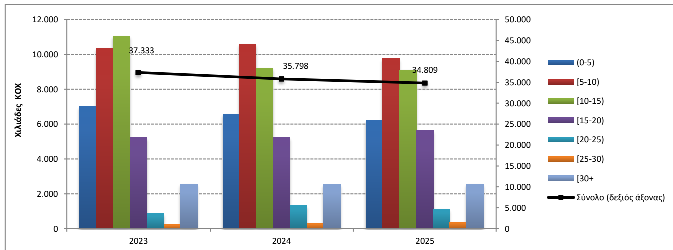
Γράφημα 4β: Κατανομή χωρητικότητας των ελληνικών εμπορικών πλοίων 100 ΚΟΧ και άνω, κατά ομάδες ηλικιών, Νοέμβριος 2023 – 2025
