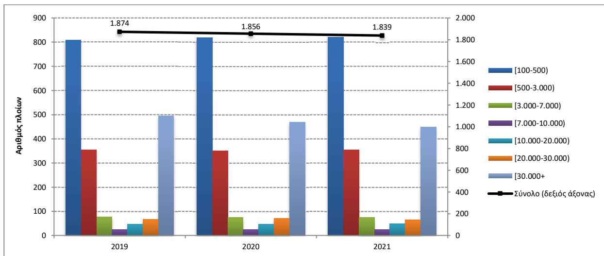
Γράφημα 3: Κατανομή των ελληνικών εμπορικών πλοίων 100 ΚΟΧ και άνω, κατά κλιμάκια ολικής χωρητικότητας, Απρίλιος 2019 – 2021
