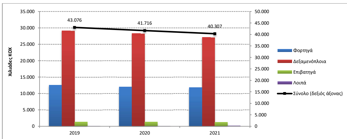
Γράφημα 2β: Χωρητικότητα των ελληνικών εμπορικών πλοίων 100 ΚΟΧ και άνω, κατά κατηγορίες πλοίων, Απρίλιος 2019 – 2021
