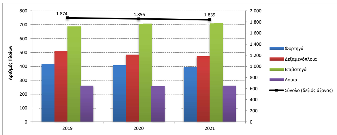
Γράφημα 2α: Δύναμη των ελληνικών εμπορικών πλοίων 100 ΚΟΧ και άνω, κατά κατηγορίες πλοίων, Απρίλιος 2019 – 2021
