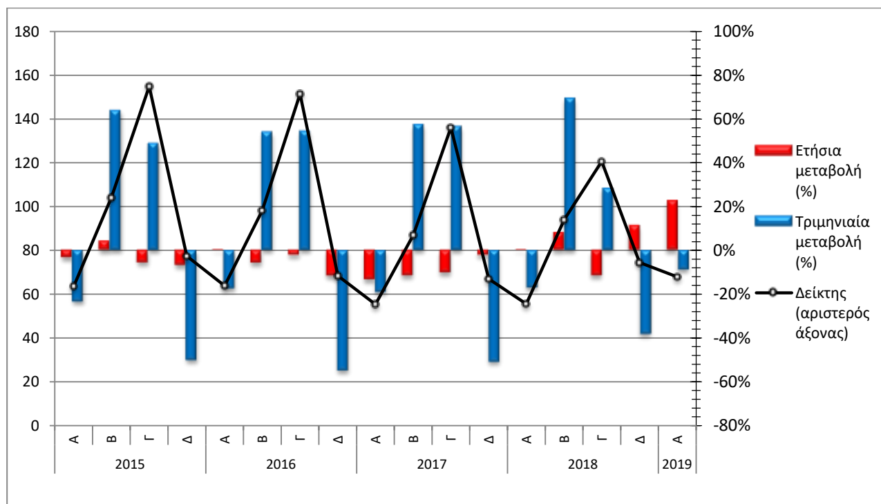
Γράφημα 2. Εξέλιξη του Δείκτη Κύκλου Εργασιών στις πλωτές μεταφορές - κλάδος 50 Nace rev.2, Έτος βάσης (2015=100,0)
