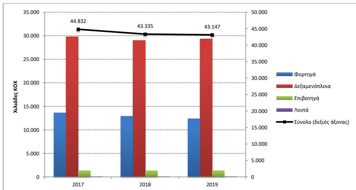
Γράφημα 2β: Χωρητικότητα των ελληνικών εμπορικών πλοίων 100 ΚΟΧ και άνω, κατά κατηγορίες πλοίων, Ιούλιος 2017 – 2019
