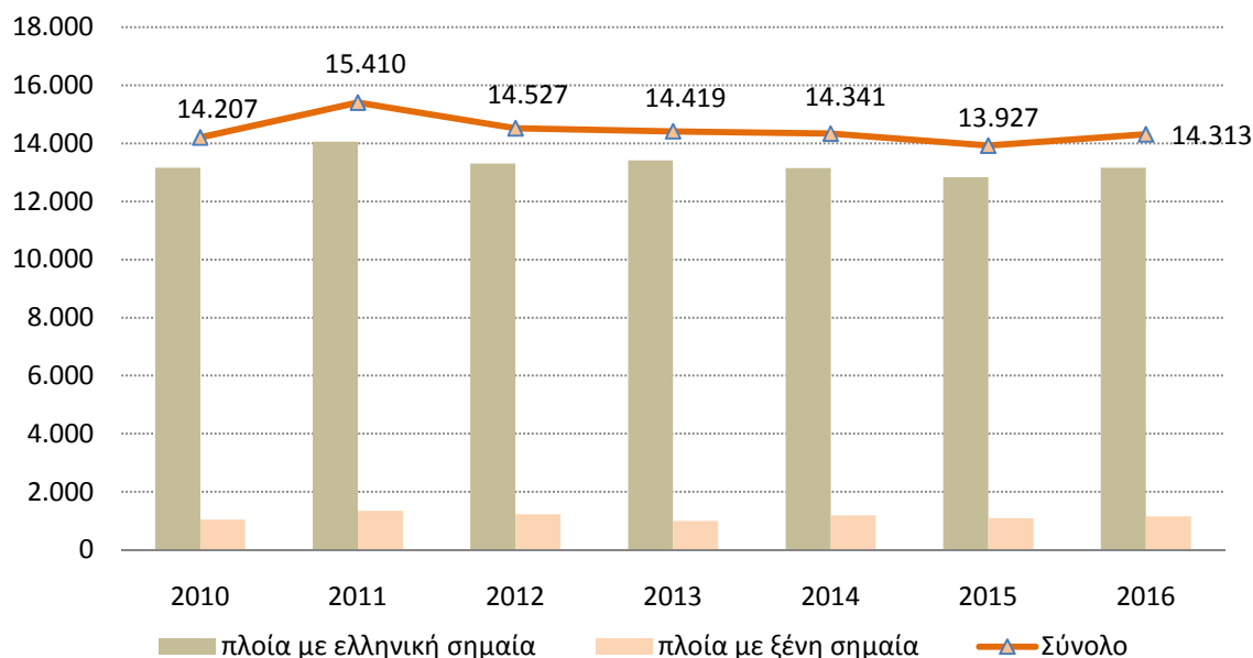
Γράφημα 1: Ναυτολογηθέντες Έλληνες ναυτικοί σε εμπορικά πλοία 100 ΚΟΧ και άνω, με ελληνική και ξένη σημαία συμβεβλημένα με το ΝΑΤ
