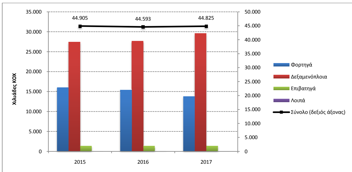
Γράφημα 2β: Χωρητικότητα των ελληνικών εμπορικών πλοίων 100 ΚΟΧ και άνω, κατά κατηγορίες πλοίων, Απρίλιος 2015 – 2017
