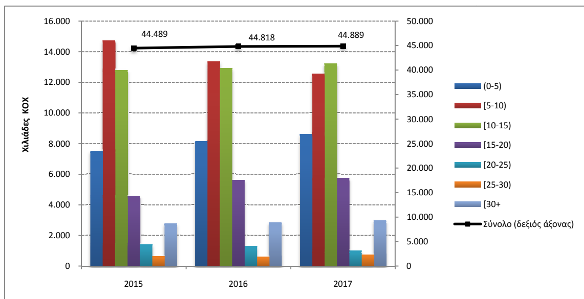
Γράφημα 4β: Κατανομή χωρητικότητας των ελληνικών εμπορικών πλοίων 100 ΚΟΧ και άνω, κατά ομάδες ηλικιών, Μάιος 2015 – 2017
