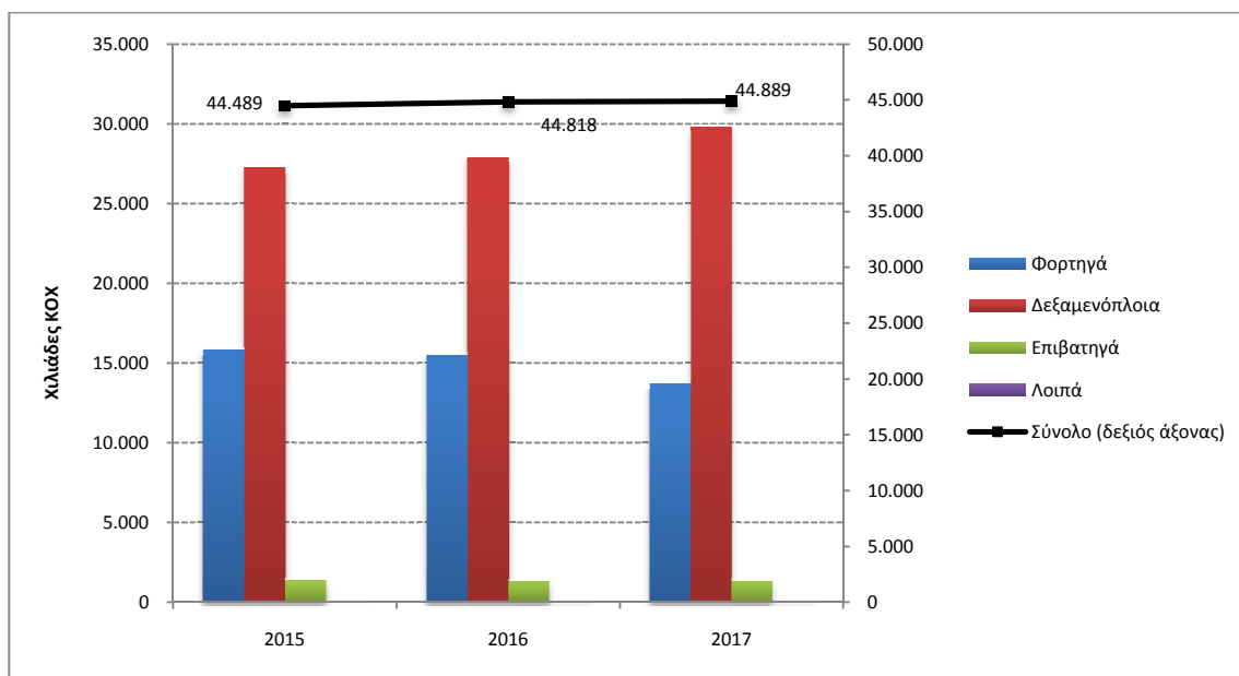
Γράφημα 2β: Χωρητικότητα των ελληνικών εμπορικών πλοίων 100 ΚΟΧ και άνω, κατά κατηγορίες πλοίων, Μάιος 2015 – 2017
