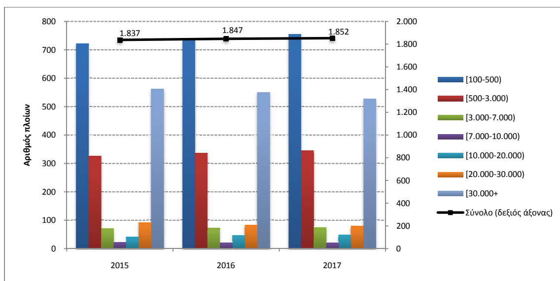
Γράφημα 3: Κατανομή των ελληνικών εμπορικών πλοίων 100 ΚΟΧ και άνω, κατά κλιμάκια ολικής χωρητικότητας, Μάιος 2015 – 2017
